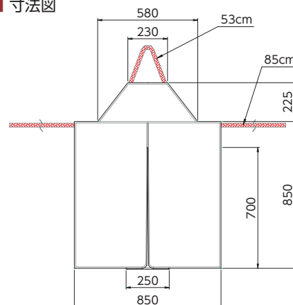
■ 寸法図
