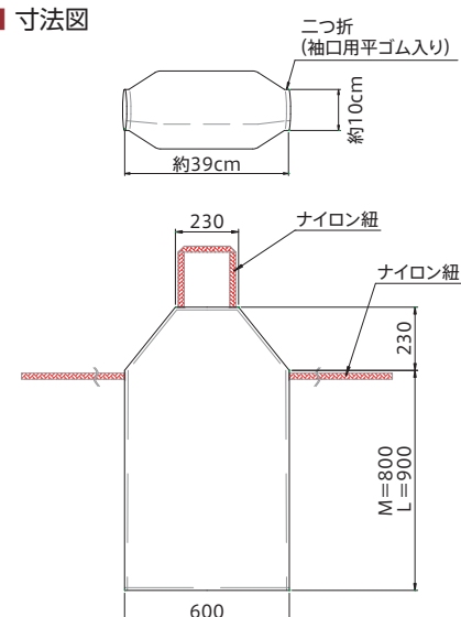
■ 寸法図
